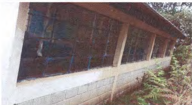
Foto1: Sustitución de pintura en muros externos e internos
